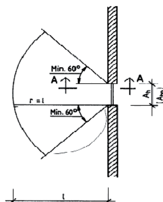
ALAPRAJZ
